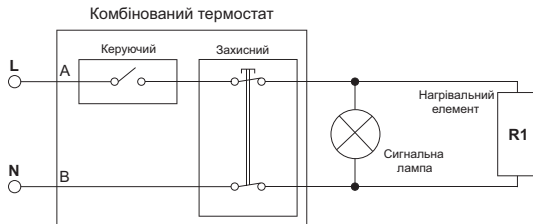
Рисунок 6. Схема електрична для моделей: N4, N4L, N4s, D400-1-M, PC, D443-1-M
