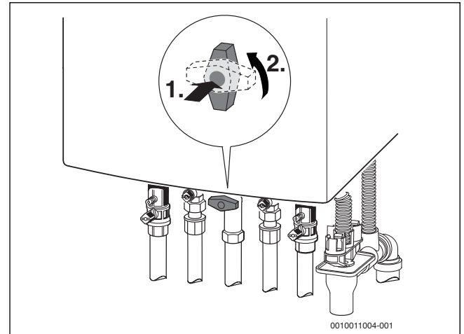
Мал. 2 Відкриття газового крана
