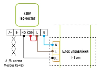
в) Схема підключення до блоку керування
