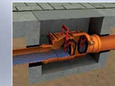
Заблокированный клапан - двойная защита от подпора.
