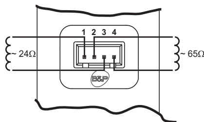
мал. 30 - Підключення газового клапану
