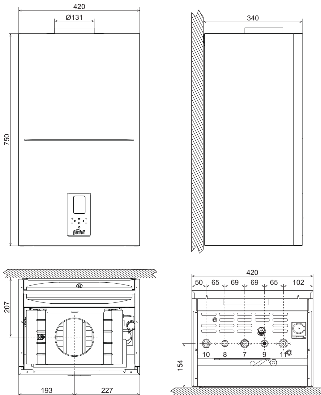
мал. 33- Розміри та під'єднувальні розміри моделі DIVATOP D C24
