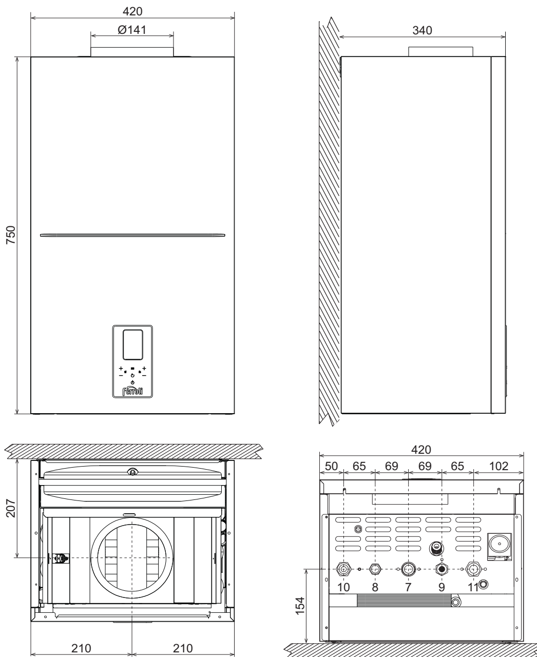
мал. 34- Розміри та під'єднувальні розміри моделі DIVATOP D C32
