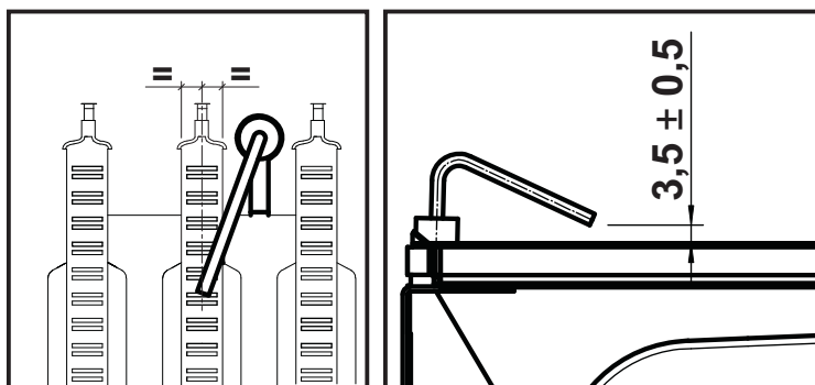
мал. 32- Розташування електрода
