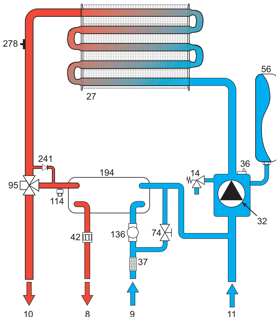
мал. 36- Контур опалення
