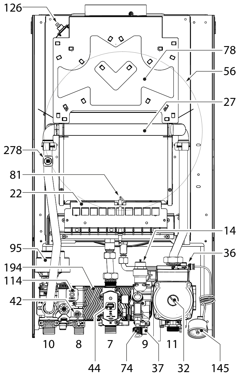
мал. 35- Загальний вигляд - DIVATOP D C24
