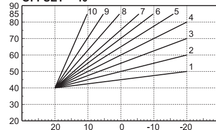
мал. 23- Пиклад паралельного пересування компенсаційних кривих
