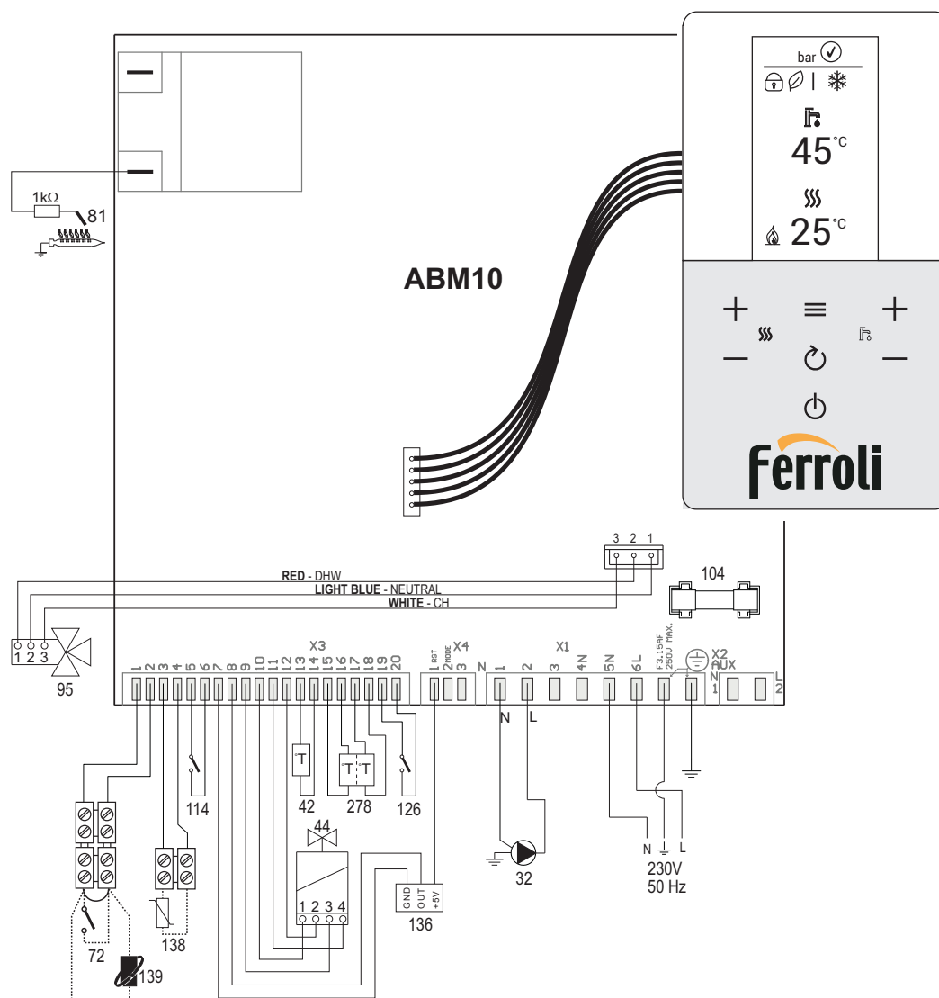
мал. 39- Електрична схема
