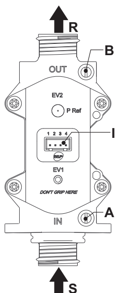
мал. 29 - Газовий вентиль
