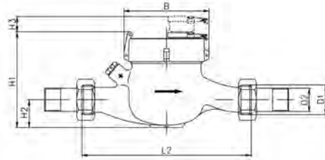
Рис. 2 Креслення лічильників води MNK
